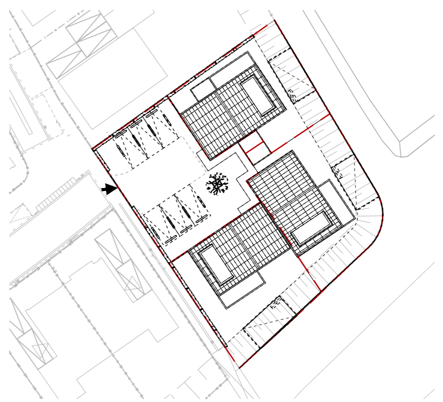
dakaanzicht schaal 1:500
